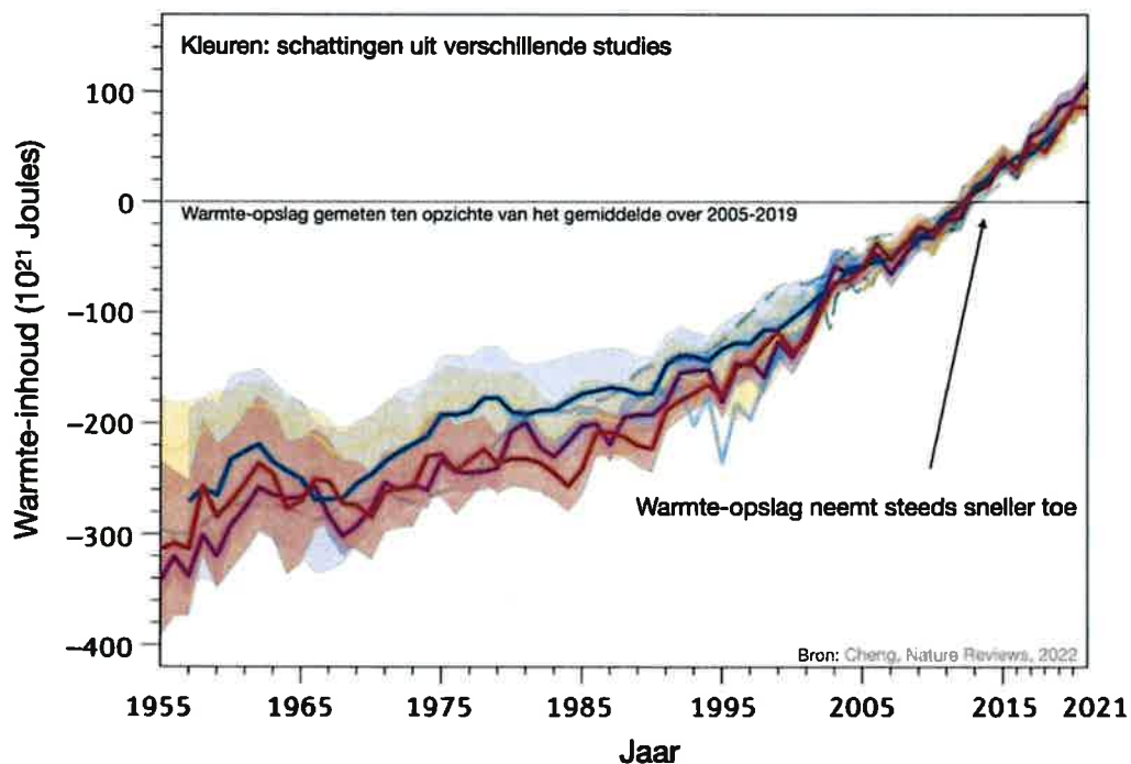
De warmte-opslag in de bovenste 2000 meter van de oceaan 1955-2021
